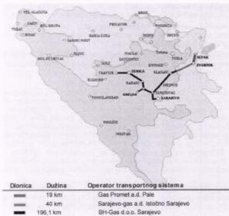
Dijagram broj 1. Transportni gasni sistem Bosne i Hercegovine
