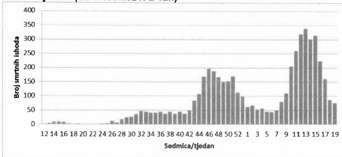
Grafikon 4. Distribucija smrtnih slučajeva od COVID-19 po tjednu, Federacija BiH (do 17.05.2021. u 12h)
