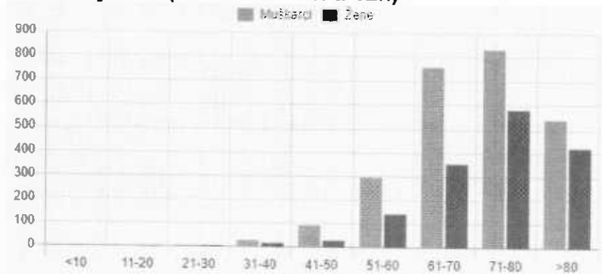
Grafikon 2. Distribucija smrtnih slučajeva od COVID-19 po dobi i spolu, Federacija BiH (do 17.05.2021. u 12h)
