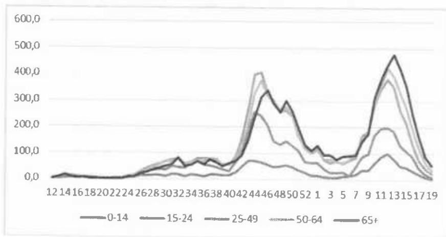
Grafikon 2. Incidenca laboratorijski potvrđenih slučajeva COVID-19 prema dobnim skupinama po tjednu, Federacija BiH 17.05.2021.
